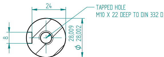
Przekrój A-A 1:1
